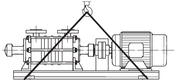
Fig. 5 Fixer l'engin de levage à l'unité de pompage avec plaque de fondation
