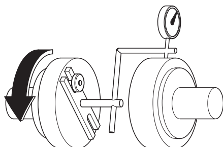
Fig. 11 Contrôle du décalage latéral et vertical
