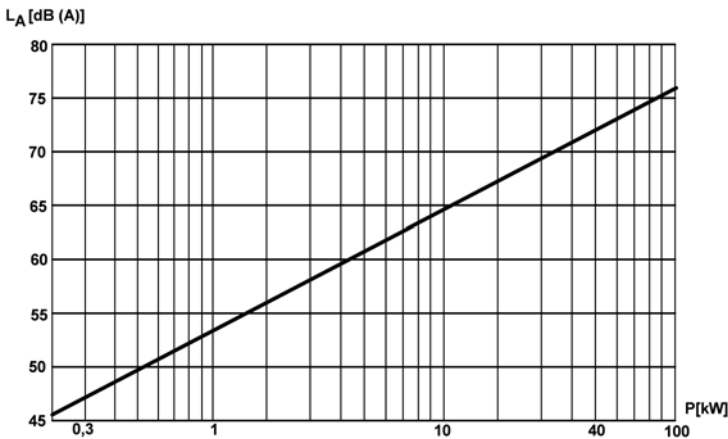
Fig. 13 Niveau de pression acoustique
