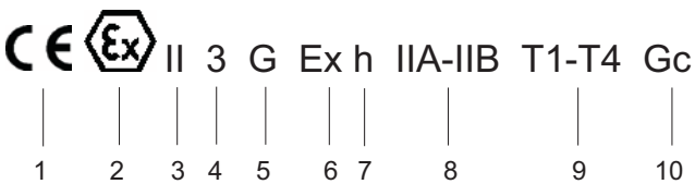
Fig. 15 Marquage relatif à la protection antidéflagrante de la pompe (groupe d'appareils II, catégorie 3)
