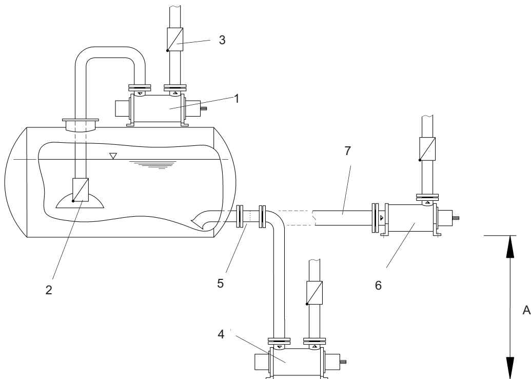
Fig. 9 Exemple de montage
