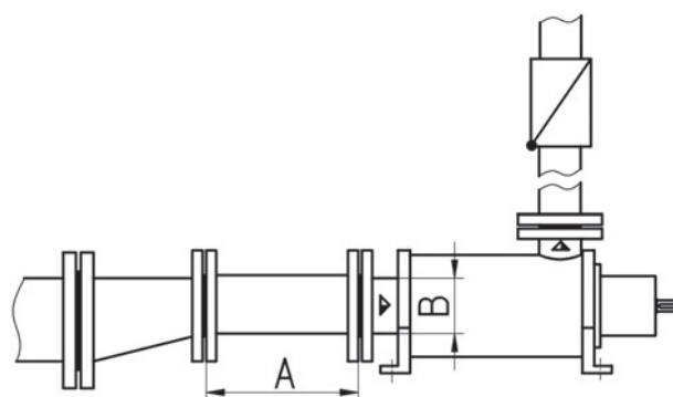
Fig. 8 Longueurs de la tuyauterie droite en amont et en aval de la pompe (recommandées)
