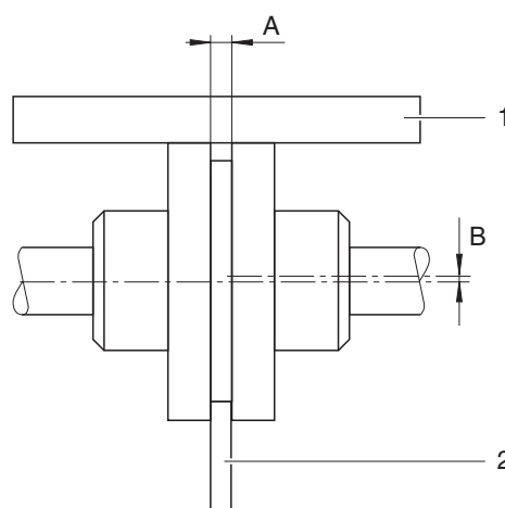
Fig. 10 Contrôle de l'alignement de l'accouplement
