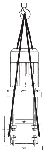
Fig. 7 Fixation de l'engin de levage au bloc-pompe (modèle vertical)
