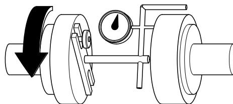
Fig. 12 Contrôle du décalage angulaire
