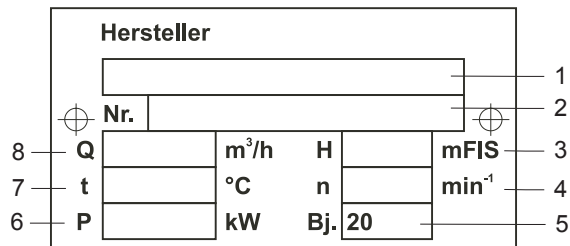
Abb. 1 Typenschild (Beispiel)
