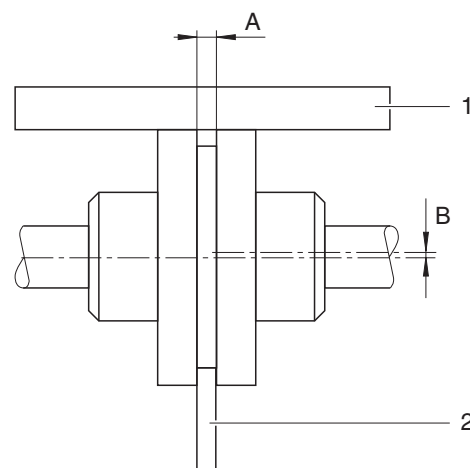
Abb. 10 Kupplungsausrichtung prüfen
