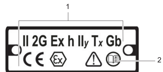
Abb. 2 ATEX-Schild (Beispiel)
