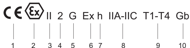
Abb. 14 Explosionsschutz-Kennzeichnung an der Pumpe (Gerätegruppe II, Kategorie 2)
