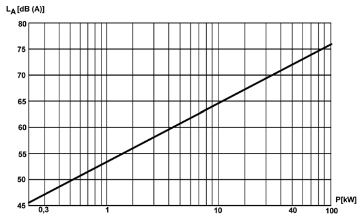
Abb. 13 Schalldruckpegel
