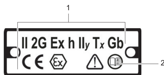
Afb. 2 ATEX-plaatje (voorbeeld)
