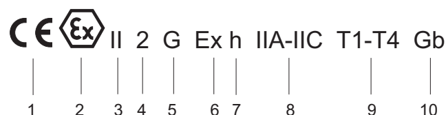
Fig. 14 Identificador de protección antiexplosión en la bomba (grupo de aparatos II, categoría 2)
