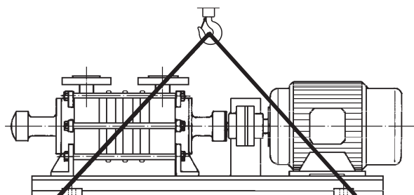
Fig. 5 Fijar el medio de elevación a grupo de bombeo con placa de base
