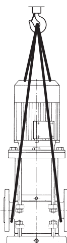
Fig. 7 Fastgørelse af løftegrej på blokpumpe (vertikal udførelse)
